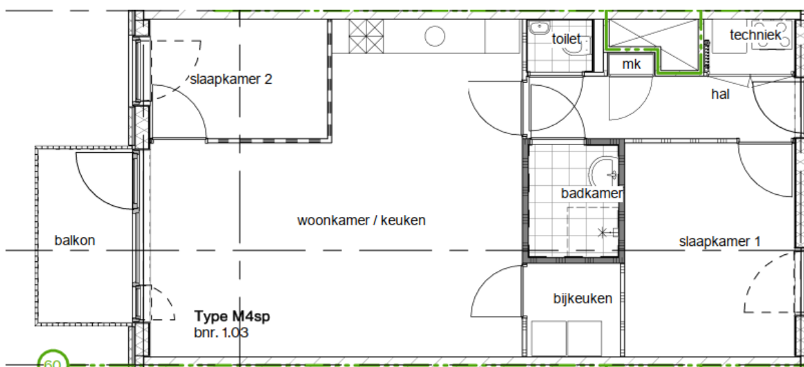
Basis plattegrond
